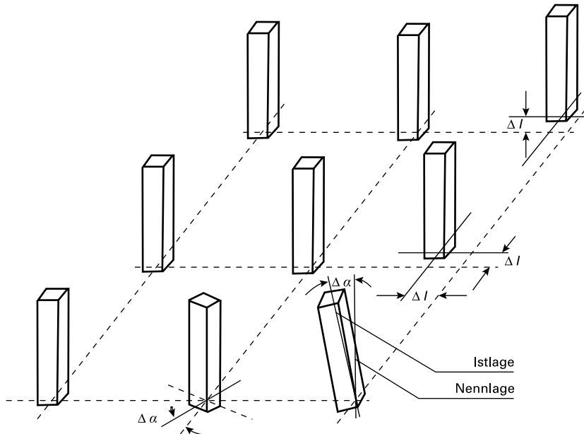
Figur 5 Lageabweichung von Bauteilen in Bauwerken von der Nennlage. Dabei kann es sich um horizontale und/oder vertikale Verschiebungen \Delta l , um Verdrehungen \Delta \alpha oder um Neigungsabweichungen \Delta \alpha , sowohl des Bauteils als auch des Achssystems, handeln.
