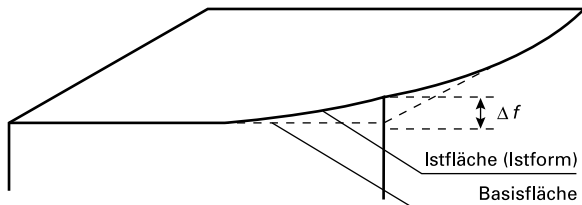
Figur 9 Massabweichungen einer Linie oder Fläche von der Sollform. Als Bezugsfläche kann z.B. eine Ebene, gegeben durch drei Punkte der Istfläche (in der Regel drei Eckpunkte), dienen
